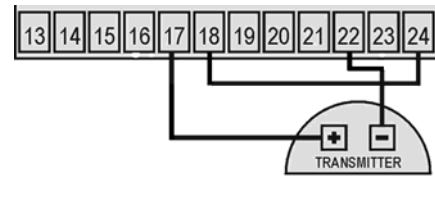
Figure 7 - Transmetteur 2 fils avec alimentation interne
