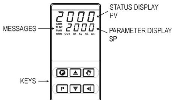
Figure 1 - Face avant
